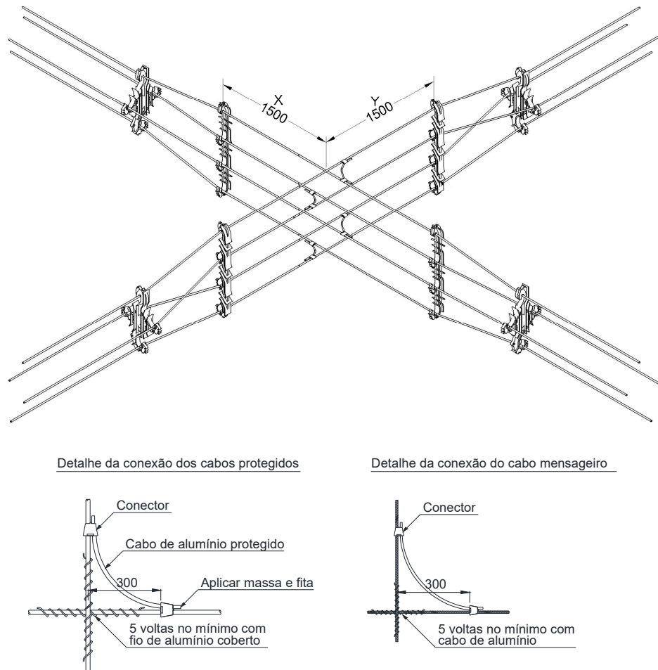
Figura 96 – Amarrações e ligações – Cruzamento aéreo
