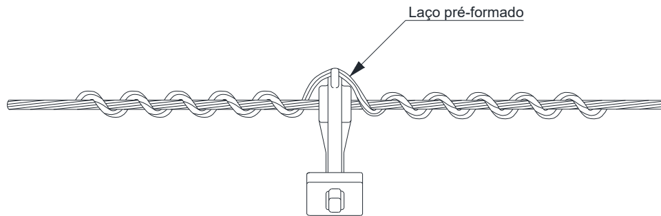
Figura 95 – Amarrações e ligações – Amarração do espaçador monofásico, vertical e losangular em cordoalha – Laço pré-formado
