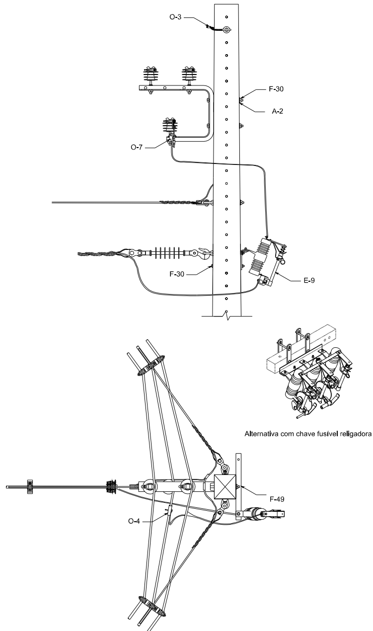
Figura 53 – Instalação de equipamento – Chave fusível em derivação monofásica – Estrutura trifásica
