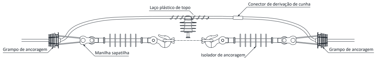
Figura 81 – Amarrações e ligações – Ancoragem dupla – Cabo protegido
