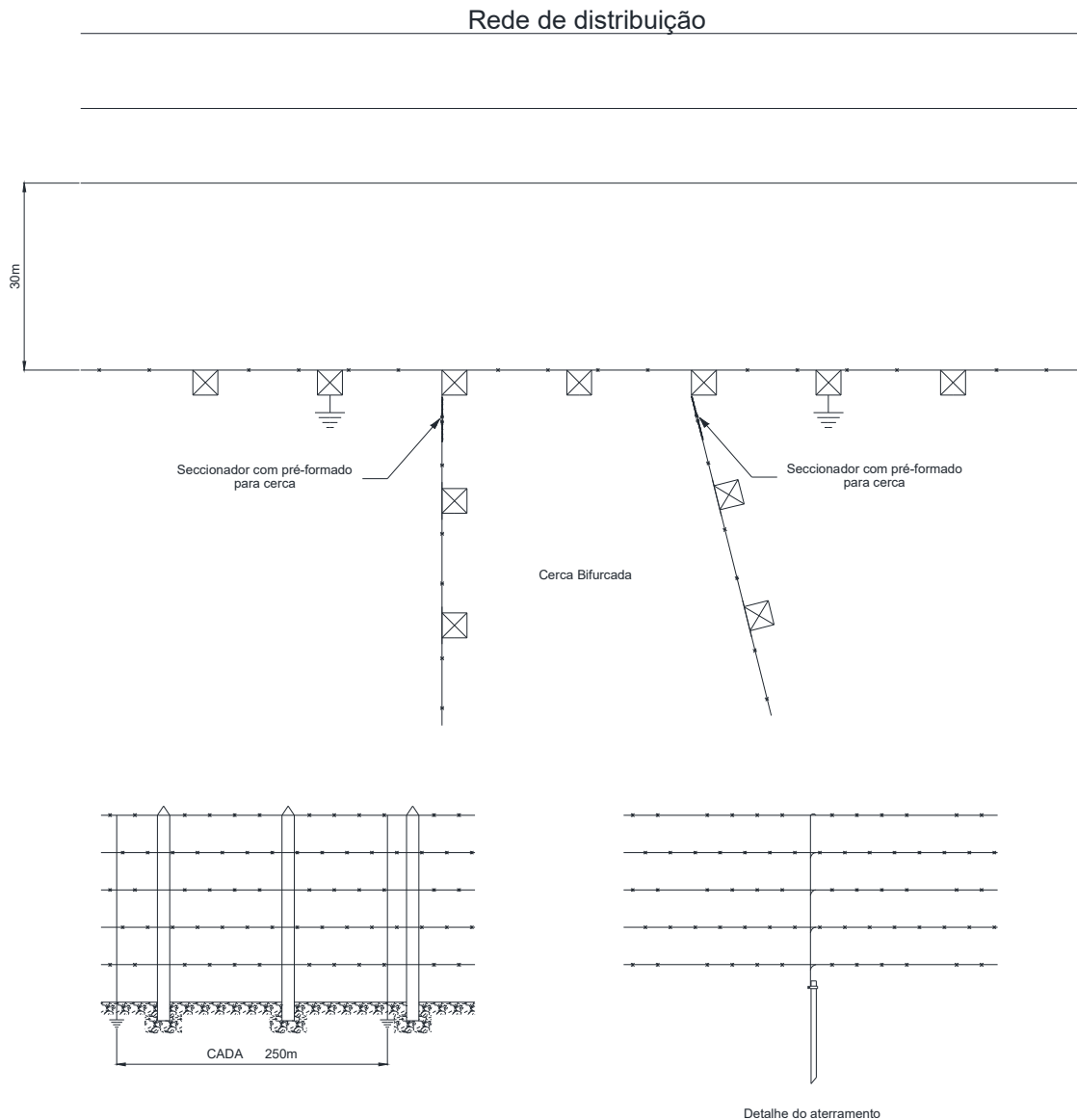
Figura 64 – Seccionamento de cerca – Cercas transversais
