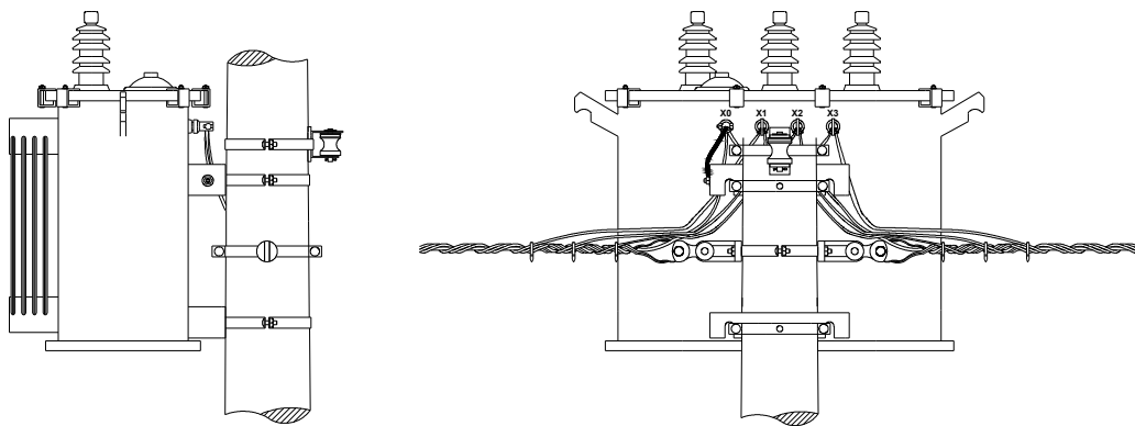
Figura 47 – Instalação de transformador – Barramento duplo
