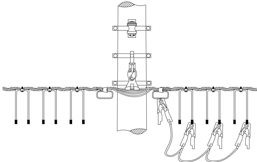
Figura 33 – Aterramento de equipamento – Aterramento temporário com garra
