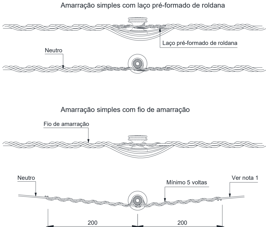
Figura 39 – Amarrações e ligações – Estrutura secundária – Tangente
