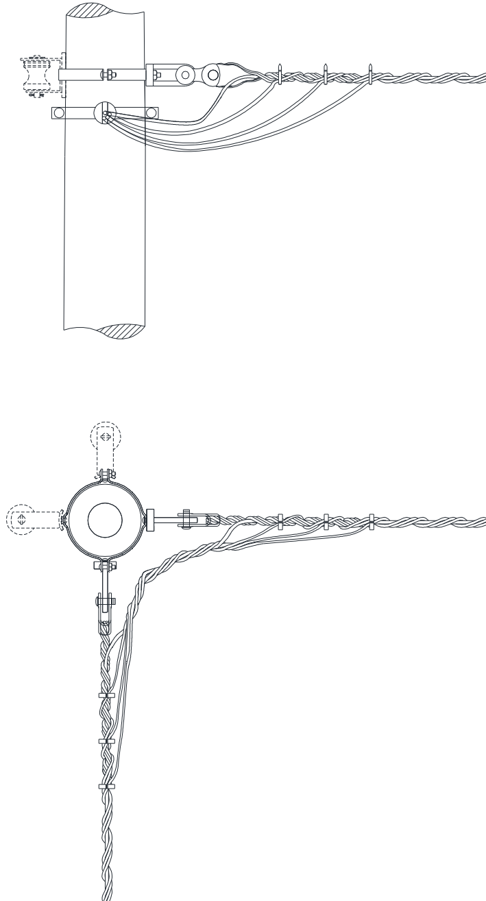
Figura 27 – Estrutura 90° - SI3 – SI3
