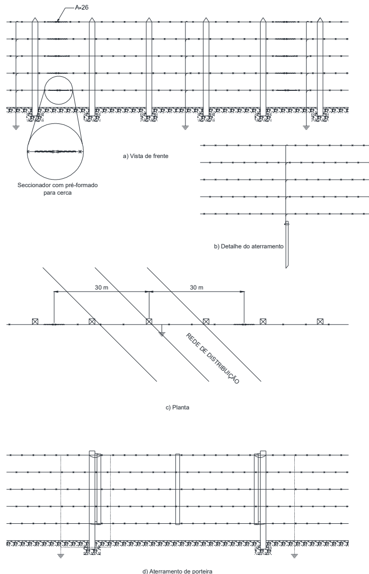
Figura 63 – Seccionamento de cerca – Cerca paralela
