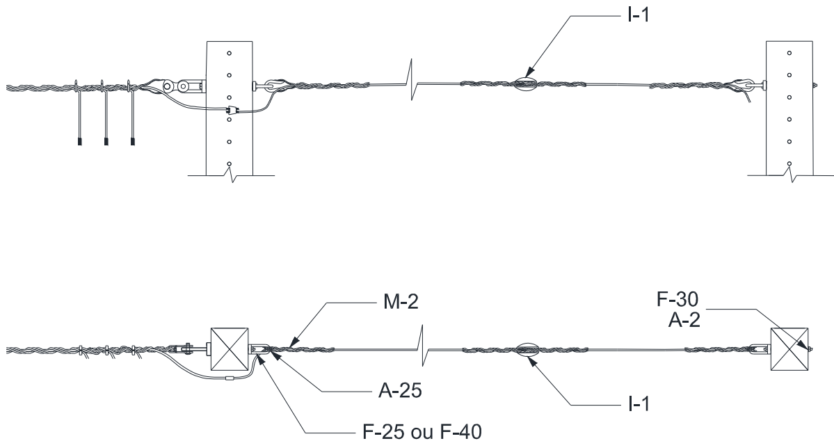
Figura 34 – Estaçamento – Estai de poste a poste
